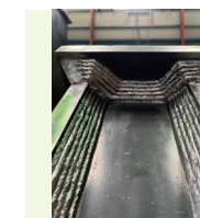
半自動溶接にて多層盛り
