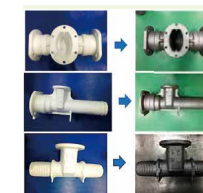
発泡模型→鋳物製品
